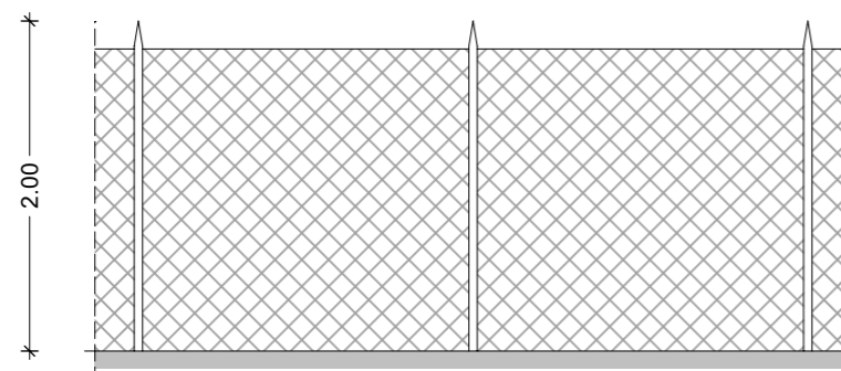
PARTICOLARE RECINZIONE
